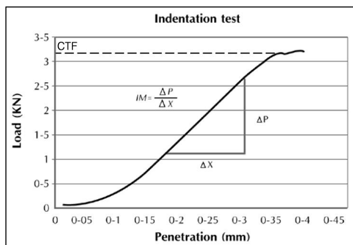
شکل ۱. نمودار شاخص مربوط به آزمایش نفوذ که در آن نحوه تعیین پارامترهای مقاومتی (CTF و IM) خرد ذرات آزمایش شده نشان داده شده است [۲۱]
