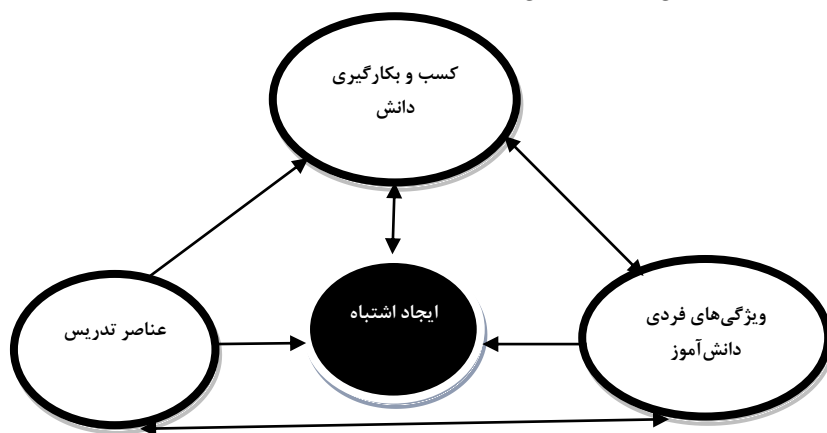
شکل ۱- مدل مربوط به روابط میان عوامل تأثیر گذار بر ایجاد اشتباهات جبری
