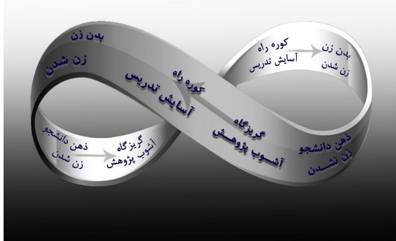
شکل ۱- دسته‌های دوتایی مضامین بر روی نوار موبیس
